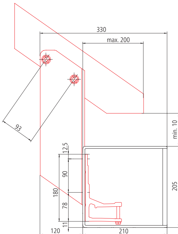
Dachsparrenhalter mit Montageplatte weinor empfiehlt den Einsatz der Montageplatte für Dachsparrenhalter.
