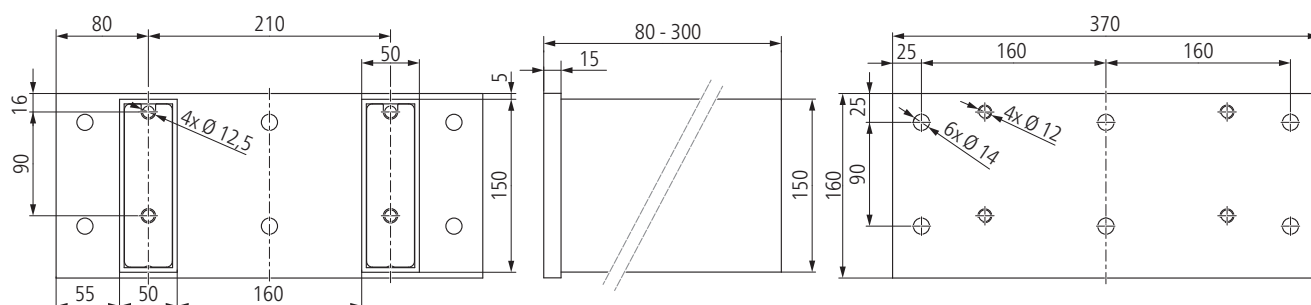
Distanzkonsole für zwei Wandkonsolen 85 mm oder einer Wandkonsole 260 mm
