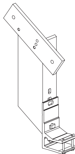
Dachsparrenhalter mit Montageplatte weinor empfiehlt den Einsatz der Montageplatte für Dachsparrenhalter.
